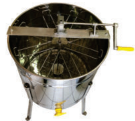
Extractor 8M A. Inox Import HE-05
